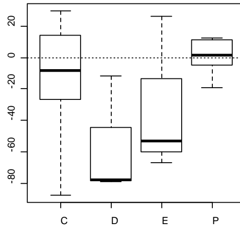
delta.pAKT
