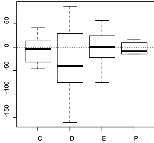
delta.pMAPK
