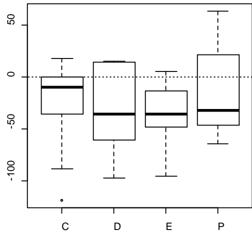
delta.pSTAT3
