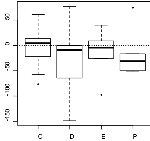
delta.pEGFR
