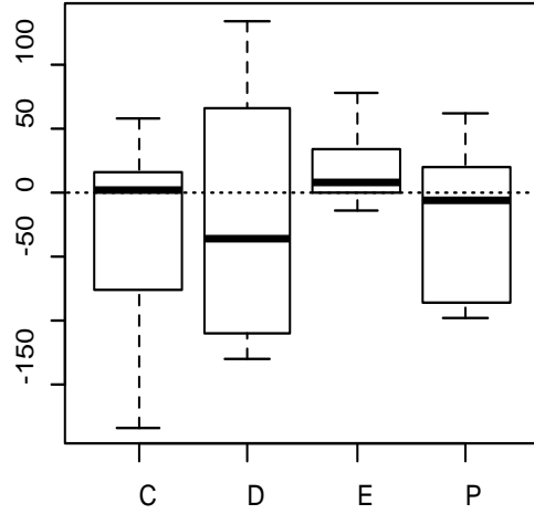
delta.Cmet
