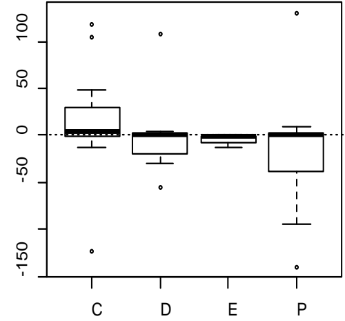
delta.Vmentin
