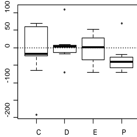
delta.EGFR
