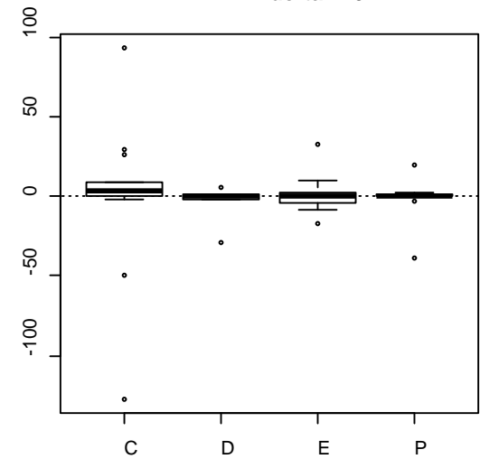
delta.IL6
