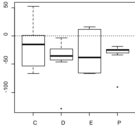
delta.pFAK
