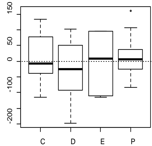
delta.Her3
