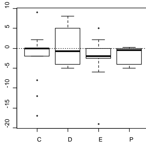
delta.TGFalpha
