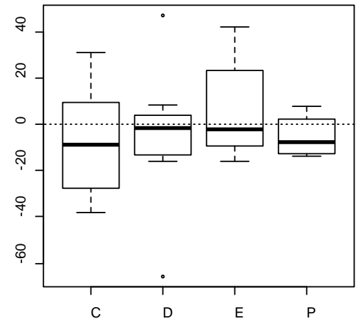
delta.pSRC
