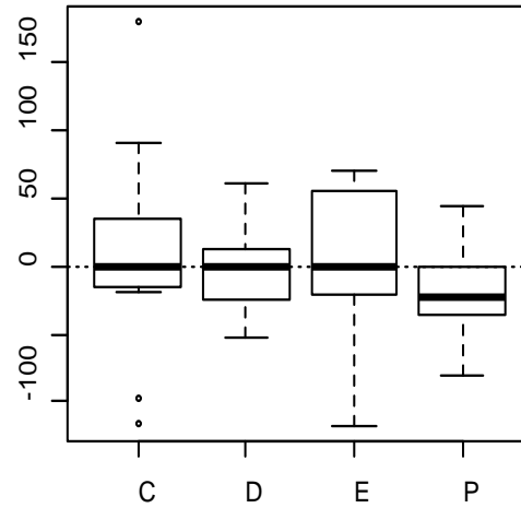
delta.Her2
