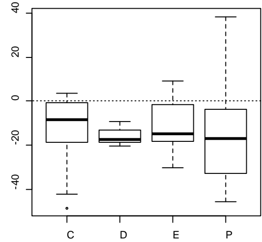
delta.pSTAT1
