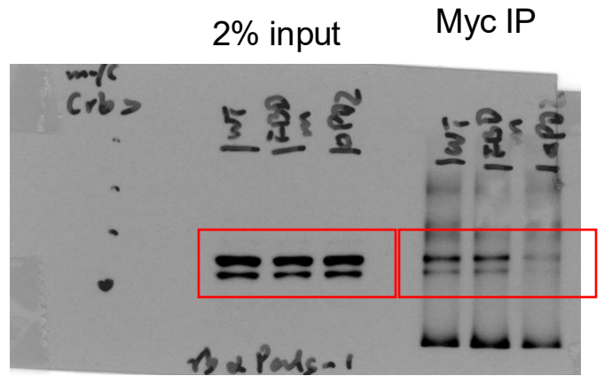
PALS1 blot
