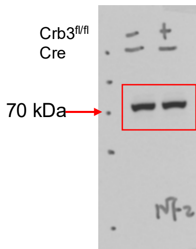
NF2 blot
