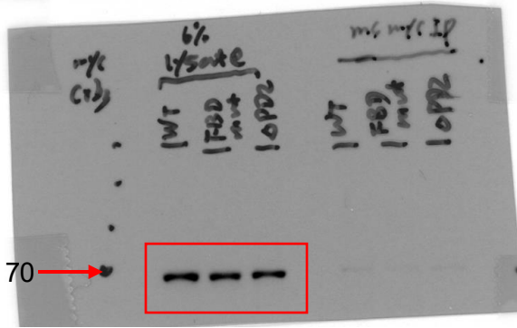
NF2 blot
