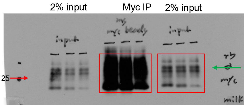
Myc blot
